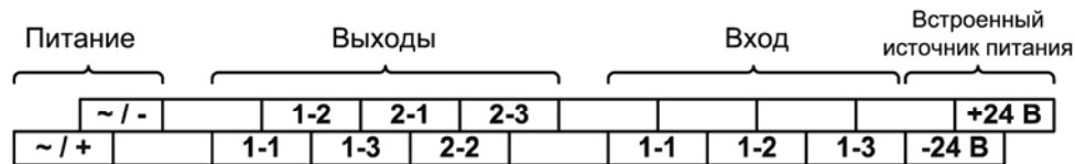
Рисунок Б.1 – Клеммная колодка прибора
