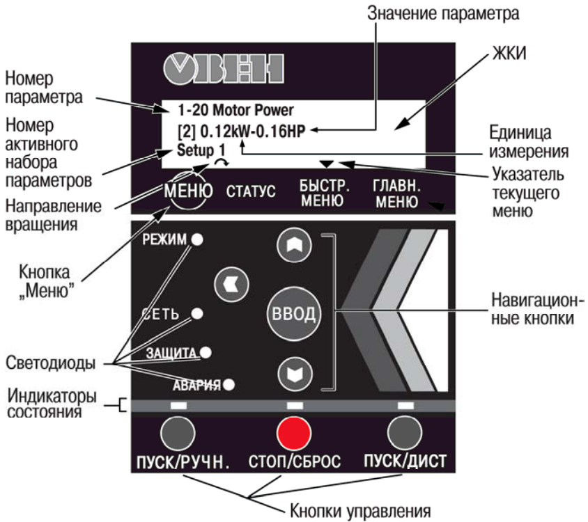
Рисунок 3.1 – ЛПО – Локальная панель оператора ПЧВ. Элементы индикации и управления
