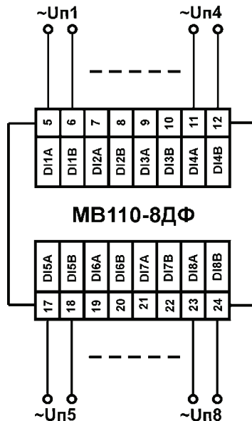
Рис. Б.2. Схема подключения к МВ110-8ДФ сигналов переменного напряжения
