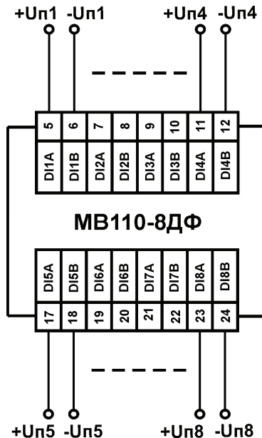
Рис. Б.3. Схема подключения к MB110-8DF сигналов постоянного напряжения
