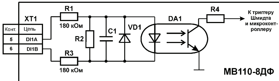
Рис. Б.5. Электрическая принципиальная схема входа MB110-8ДФ (схема других входов идентична приведенной)
