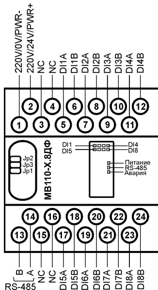
Рис. Б.1. Общий чертеж MB110
