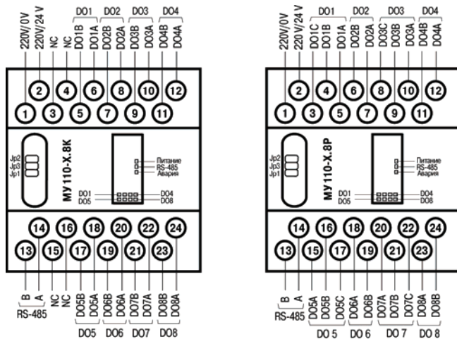
Рис. Б.1. Общий чертёж МУ110-8Р и МУ110-8К
