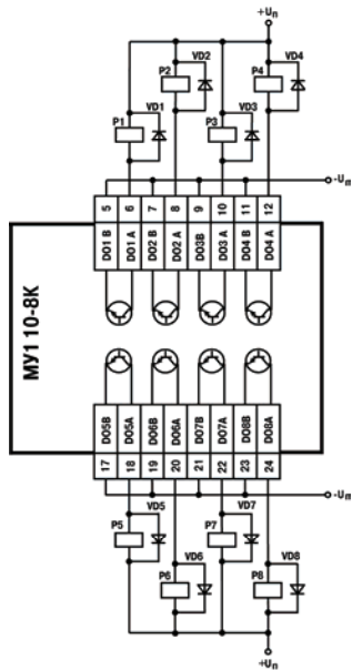
Рис. Б.3. Схема подключения нагрузки к ВЭ типа К (для МУ110-8К)
