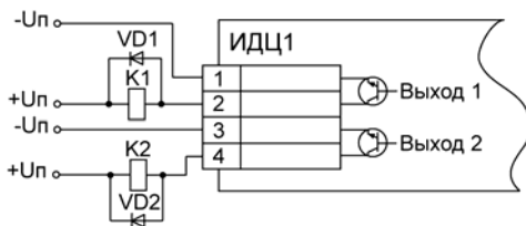
Рисунок 3.6 – Схема подключения к прибору реле
