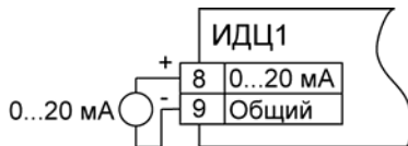
Рисунок 3.4 – Схема подключения ко входу прибора датчиков с сигналами тока от 0 до 5 мА, от 0 до 20 мА, от 4 до 20 мА
