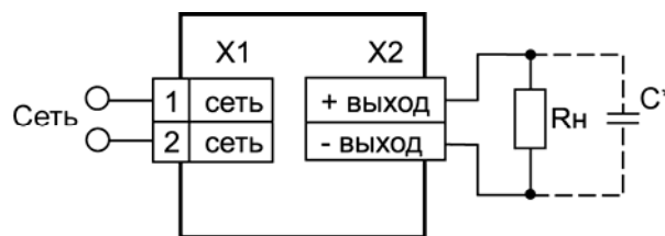
Рисунок 2 – Типовая схема подключения блока питания БП15Б-Д2-х
