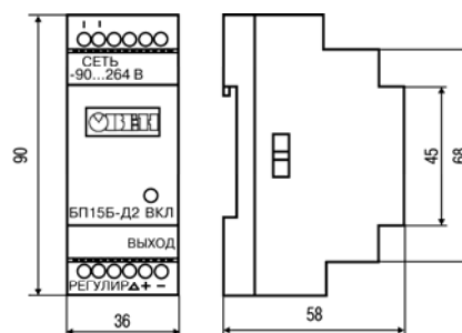
Рисунок 1 – Габаритные размеры блока питания БП15Б-Д2-х
