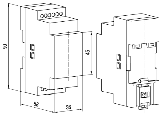
Рисунок 1 – Габаритный чертеж блока
