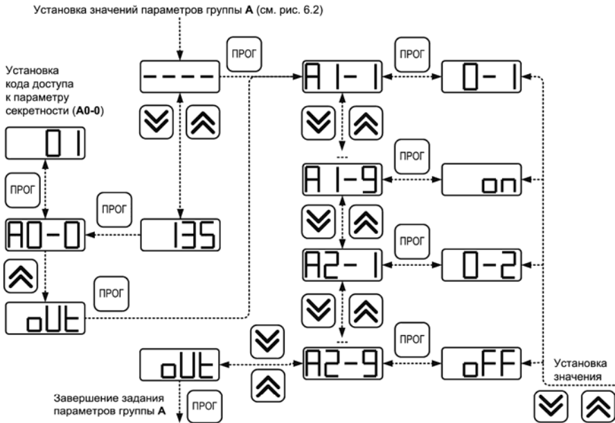
Рисунок 6.3 – Последовательность работы с прибором на втором уровне программирования для группы параметров «А»
