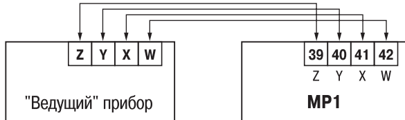
Рис. Б8. Схема подключения модуля к «ведущему» прибору
