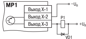
Рис. Б3. Схема подключения силового реле к выходному элементу типа K (транзисторная оптопара n-p-n-типа)
