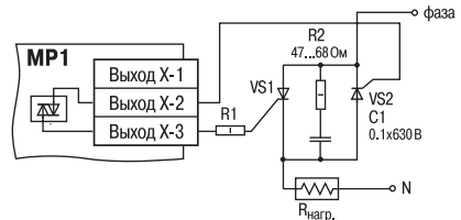
Рис. Б5. Схема подключения двух силовых тиристоров к ВЭ типа С (симисторная оптопара)
