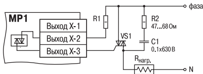
Рис. Б4. Схема подключения силового симистора к ВЭ типа С (симисторная оптопара)
