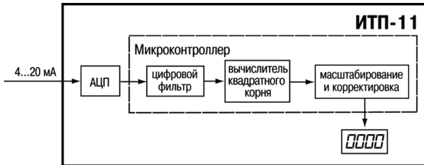
Рисунок 3.1 – Структурная схема прибора
