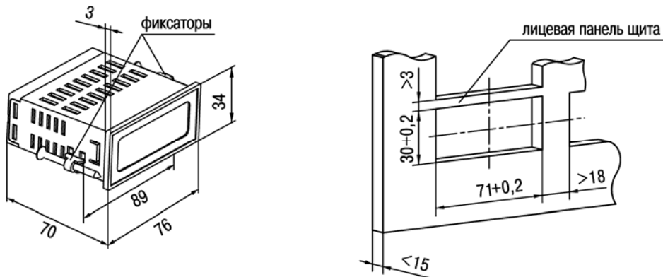
Рисунок А.1 – Габаритный чертеж прибора в корпусе ЩЗ
