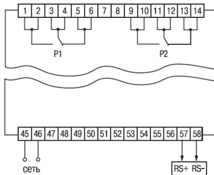
Рис. Б.5. Подключение выходных реле
