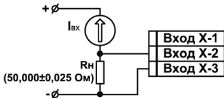
Рисунок Б.12 – Схема подключения активного датчика с токовым выходом 0... 5, 0... 20 или 4... 20 мА
