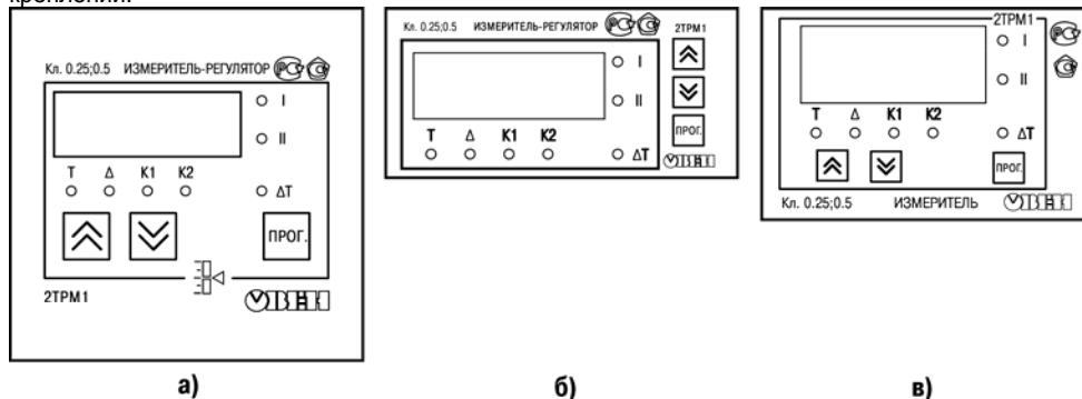
Рисунок 3.5 – Лицевая панель прибора для корпусов: а) настенного Н и щитового крепления Щ1; б) – щитового Щ2; в) – DIN-реечного Д
