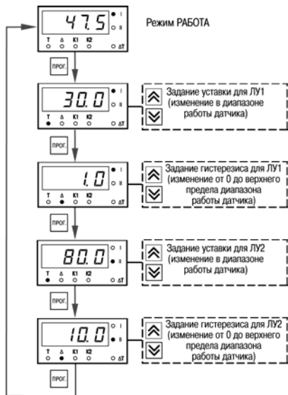
Рисунок 6.1 – Последовательность работы с прибором на первом уровне программирования
