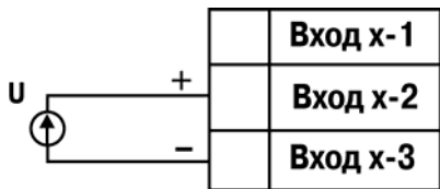
Рисунок Б.10 – Схема подключения активного датчика с выходом в виде напряжения -50...50 мВ или 0...1 В
